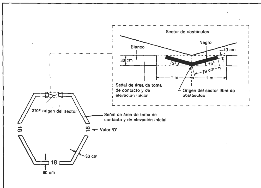
Figura 5-5H. Señal de sector despejado de obstáculos de heliplateforma
