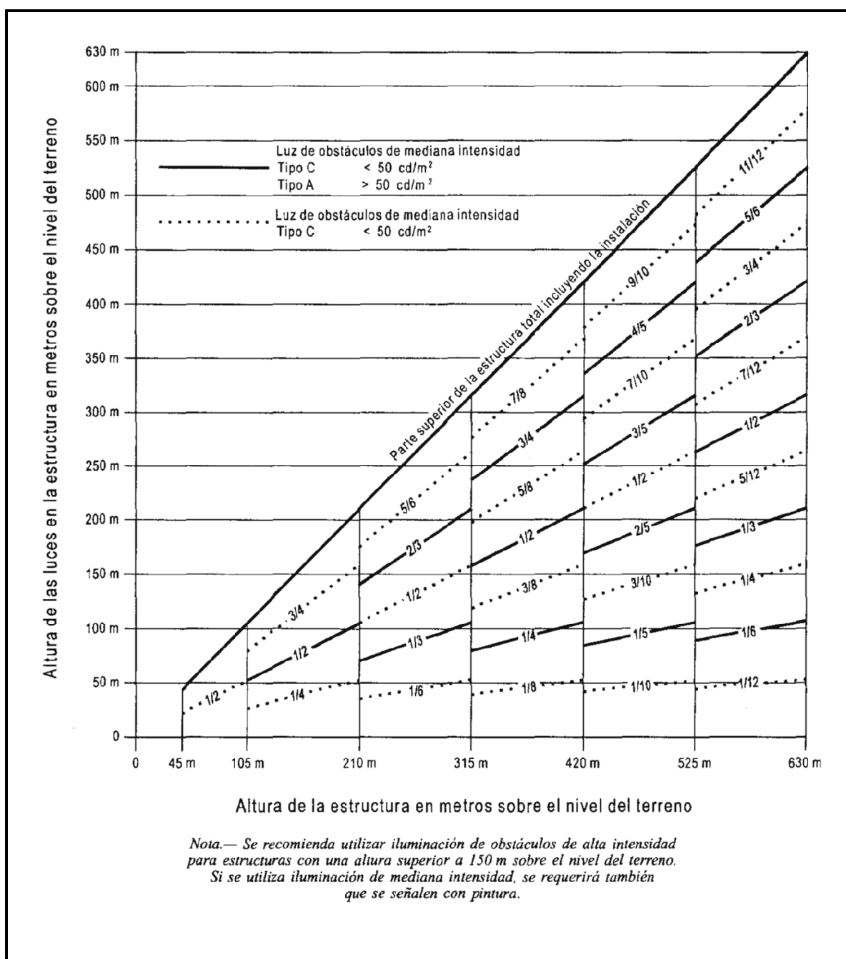
Figura A6 – 5. Sistema doble de iluminación de obstáculos de mediana intensidad de Tipo A / Tipo C
