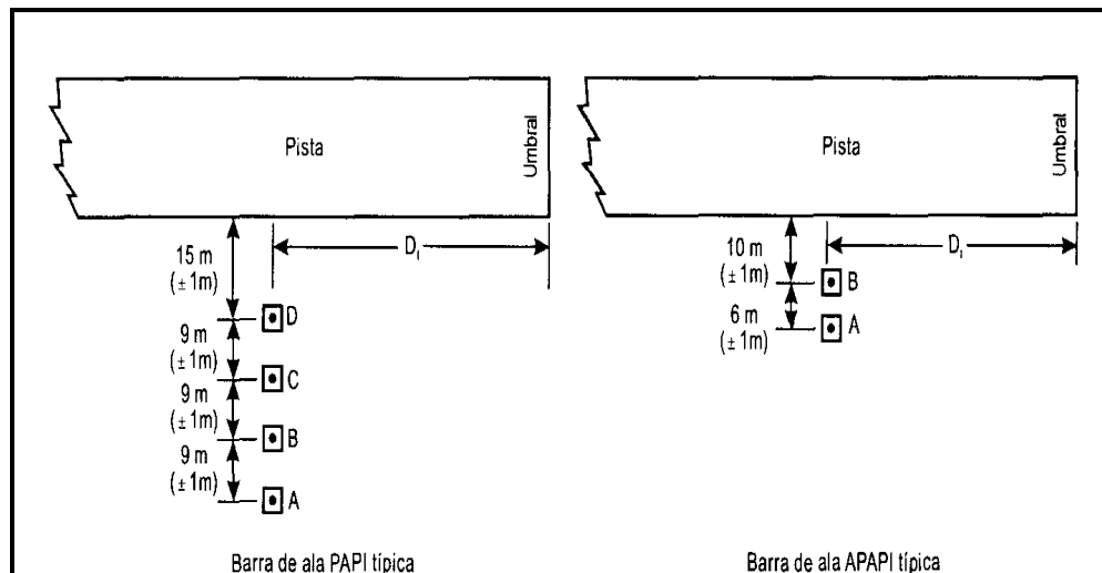
Figura 5-18. Emplazamiento del PAPI y del APAPI
